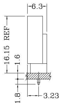
S-Type/直插型
