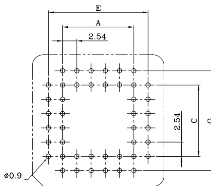
PCB LAYOUT 线路板布局图
