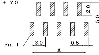
PCB LAYOUT (TYPE-A) 线路板布局图 (正脚位)
