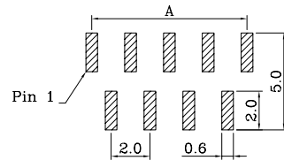
PCB LAYOUT (TYPE-B) 线路板布局图 (反脚位)
