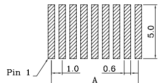
PCB LAYOUT (TYPE-D) 线路板布局图 (并脚位)
