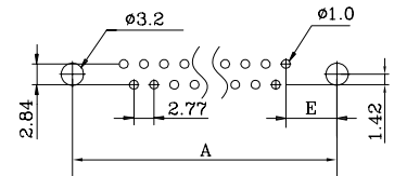
PCB LAYOUT 线路板布局图
