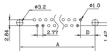
PCB LAYOUT 线路板布局图
