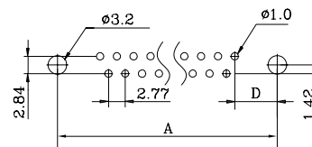
PCB LAYOUT 线路板布局图
