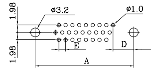
PCB LAYOUT 线路板布局图
