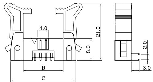
Right Angle/弯插
