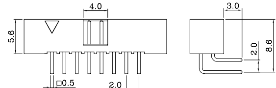
Right Angle/弯插
